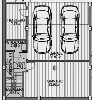
PLANTA SÓTANO
