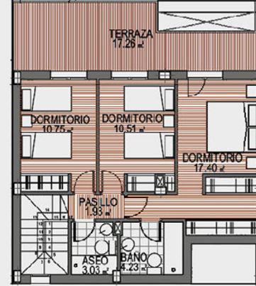
PLANTA PRIMERA
